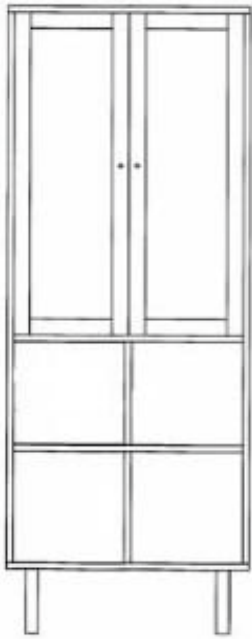
Model: 625-1 Størrelse: B75 x D40 x H195 cm
